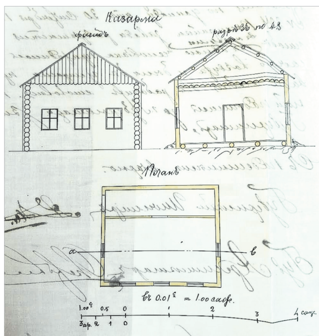
Казарма для рабочих (ГАЯО. Ф. 80. Оп. 1. Д. 1354. Л. 90б).
