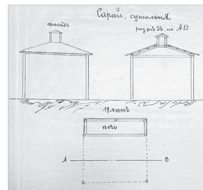
Сарай-сушильня (ГАЯО. Ф. 80. Оп. 1. Д. 1354. Л. 90б).
