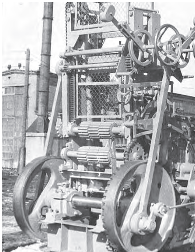
Лесопильная рама Р65-4, 1962 г.
