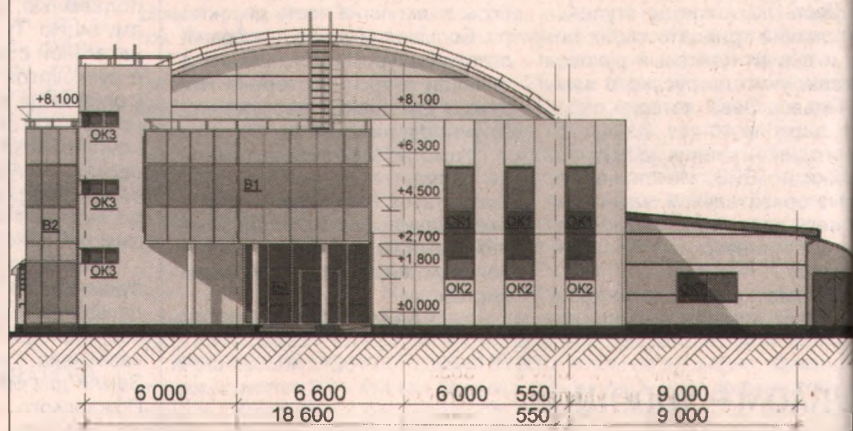
Фасад 1-4/2
